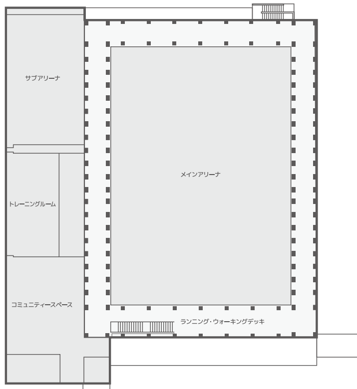
2 F 平面図
